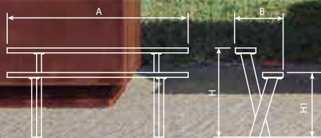
A: 1850mm B: 490mm H: 910mm H1: 660mm
